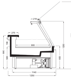
LEOPARD V1 900 IFG/SD
