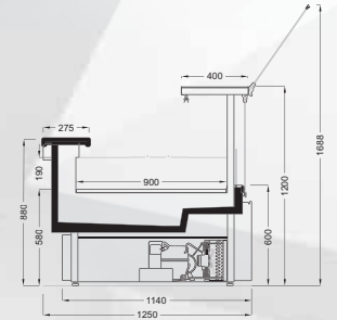
LEOPARD V1 900 FG/SD
