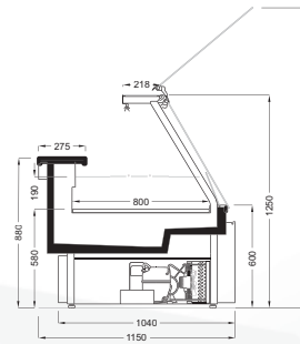
LEOPARD V1 800 IFG/SD
