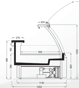
LEOPARD V1 900 CG/SD
