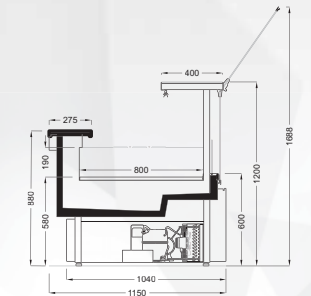
LEOPARD V1 800 FG/SD
