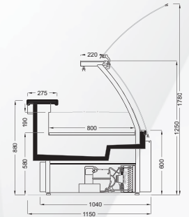
LEOPARD V1 800 CG/SD
